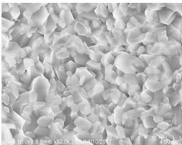
Fig.5 Images FEG de la surface du PM2000 oxydé 48h sous air à 1200°C.
