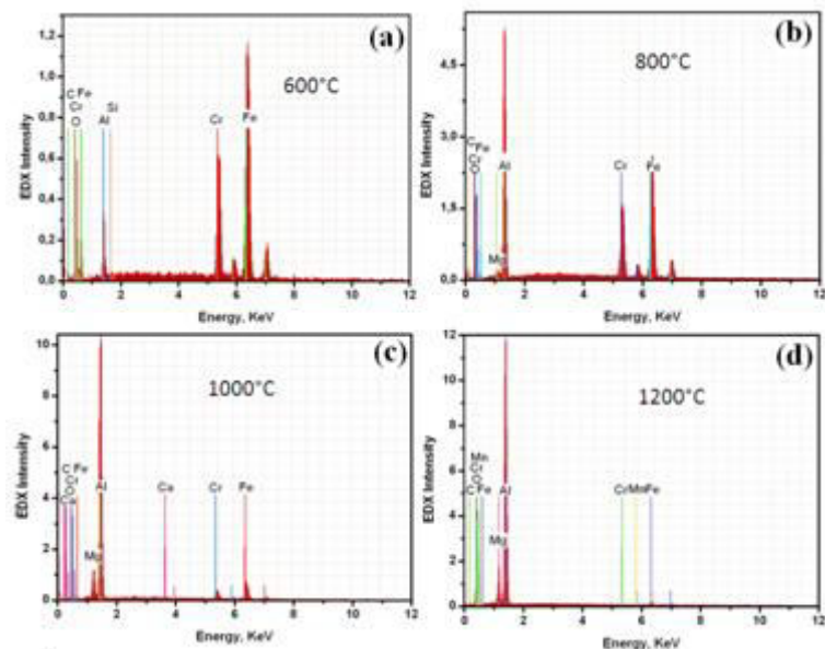
Figure 3 : Analyses EDX des divers alliages de PM2000 oxydés sous air durant 48h (a) 600°C, (b) 800°C, (c) 1000°C, et 1200°C.
