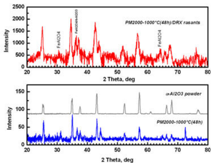
Fig.6 Spectres de diffraction des rayons X de l'alliage PM2000 oxydé à 1000°C (48h), en conditions rasantes (2.5°) en en conditions classiques (rouge et bleu respectivement), et comparaison avec un spectre de la poudre d'alumine alpha (de référence).
